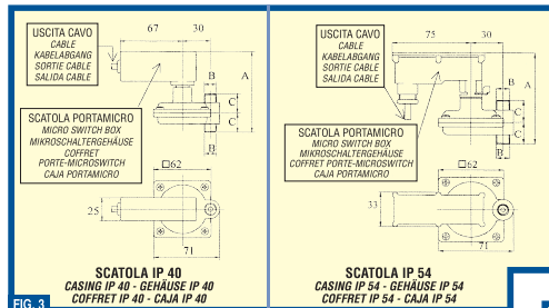
Fig. 3: Casing IP40: is connected to the pressure switch with 4 screw closure of the box. Casing IP54: is connected to the pressure switch by means of a rapid connection and seeger. Gehäuse IP54: Am Messingkörper durch das Gehäuse selbst, mittels 4 Schrauben befestigt. Gehäuse IP54: Am Messingkörper mittels Schnellverbindung und Seegering verbunden. COFFRET IP40: raccordé au pressostat par 4 vis. COFFRET IP54: raccordé au pressostat par 4 vis rapides seeger. Fig. 3: Casing IP40: conectado al presostato mediante cierre con 4 tornillos de la propia caja. CAJA IP 54: conectada al presostato mediante conexión rápida y anillo seeger.
